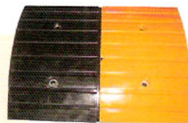
型号: CAS-LG-8(优质) 品名: 流线型减速坡 规格: 500×370×50mm 适用: 花园小区
