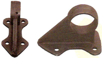
型号：CAS-DLZ-3 品名：挡轮座（四个螺丝孔）中间穿孔 规格： \phi 2.0 \setminus \phi 2.5 \setminus \phi 3.0
