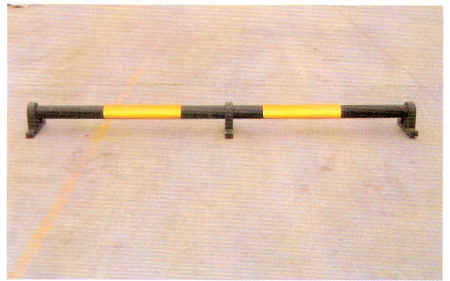
型号: CAS-DLG-2 品名: 挡轮杆 规格: \phi 2.0 \times 2000 \text{mm} \ \phi 2.5 \times 2000 \text{mm} \phi 3.0 \times 2000 \text{mm}
