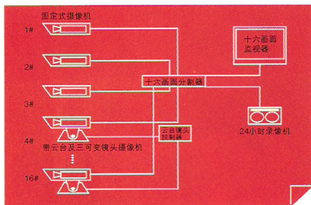
16画面监控设备结构图
