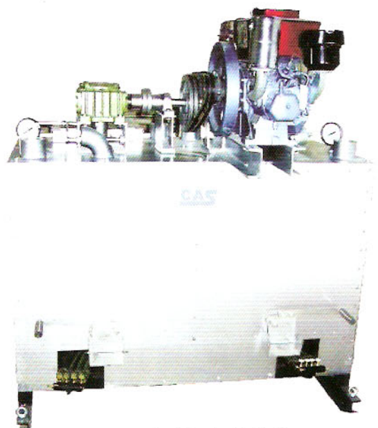
○ 机械双缸热熔釜
