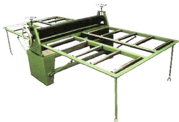
○贴膜机
