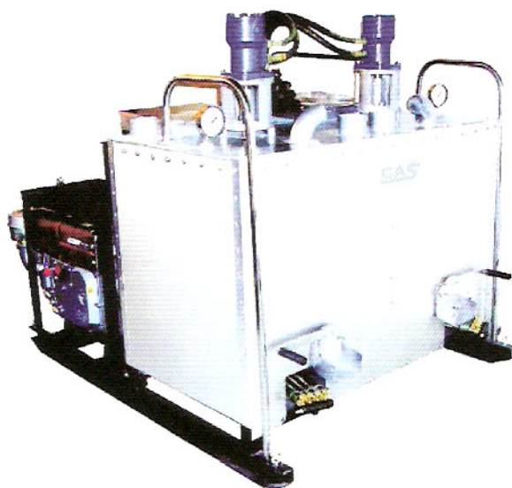
○ 液压双缸热熔釜
